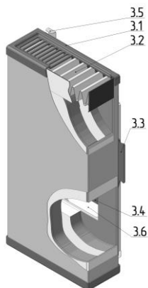
Рис. 2 Устройство шумоглушителя
